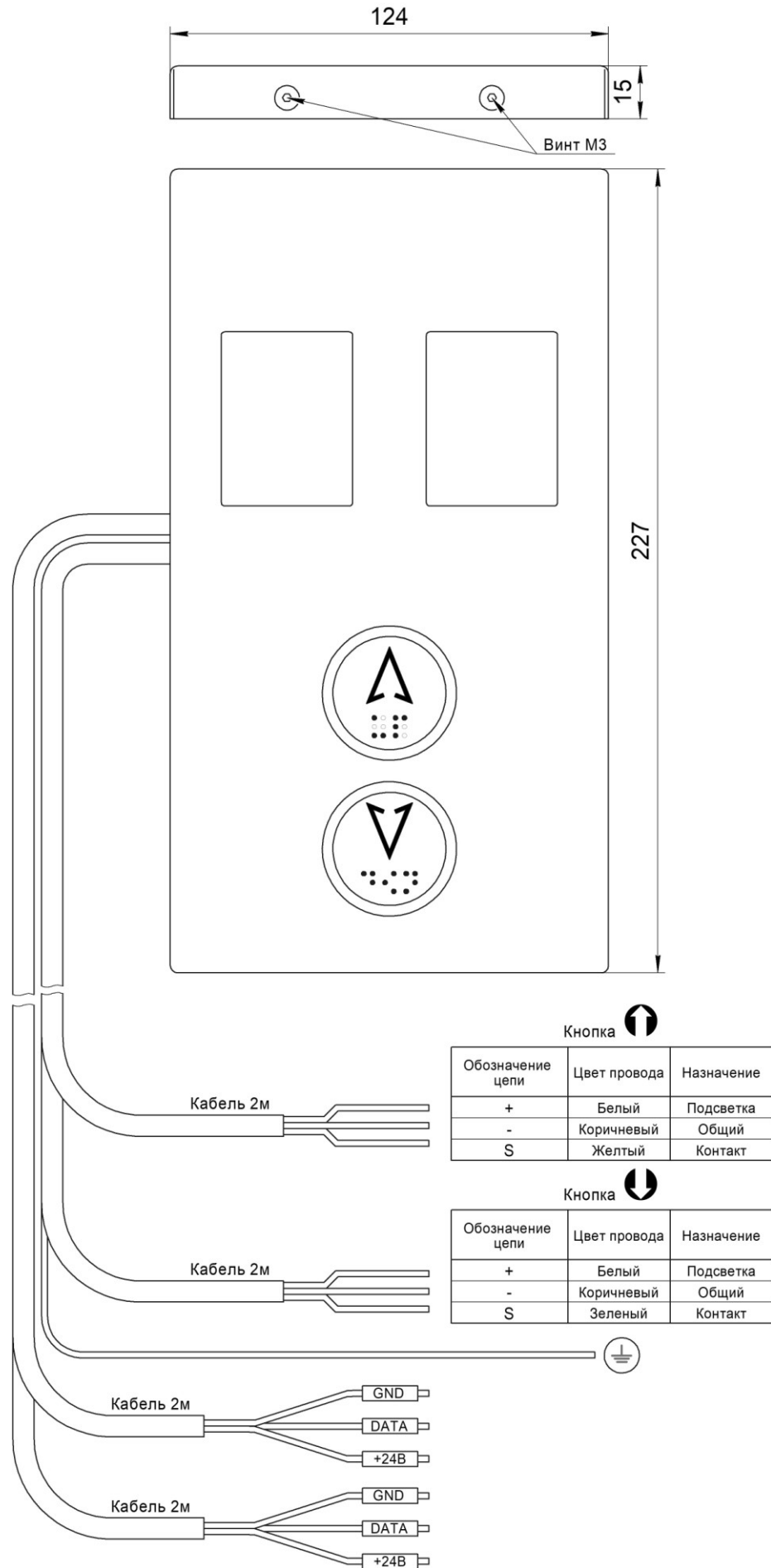
Рис.1 Внешний вид, габаритные и установочные размеры Вызывного поста КВАДРО НШЕК.468381.069
